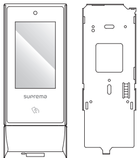
デバイスおよび壁用ブラケット (XS2-QAPB, XS2-QDPB)
