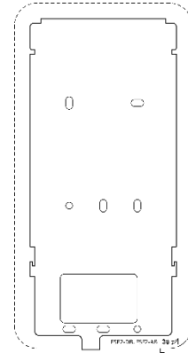
드릴링 템플릿
