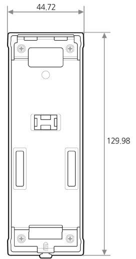
확장 브래킷
