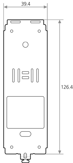
기본 브래킷
