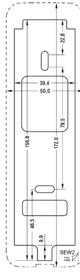
드릴링 템플릿
