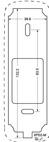
드릴링 템플릿
