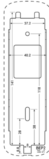
드릴링 템플릿
